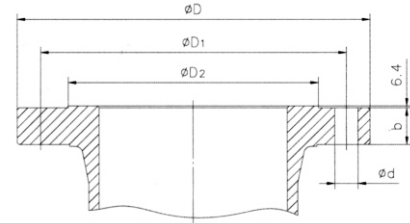
Class 600-2500LB RF 法兰/Flanges
