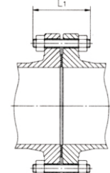
螺柱螺栓长度 Length of Stud Bolt
