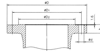
Class150LB & Class 300LB RF 法兰/Flanges
