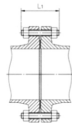
螺柱螺栓长度 Length of Stud Bolt
